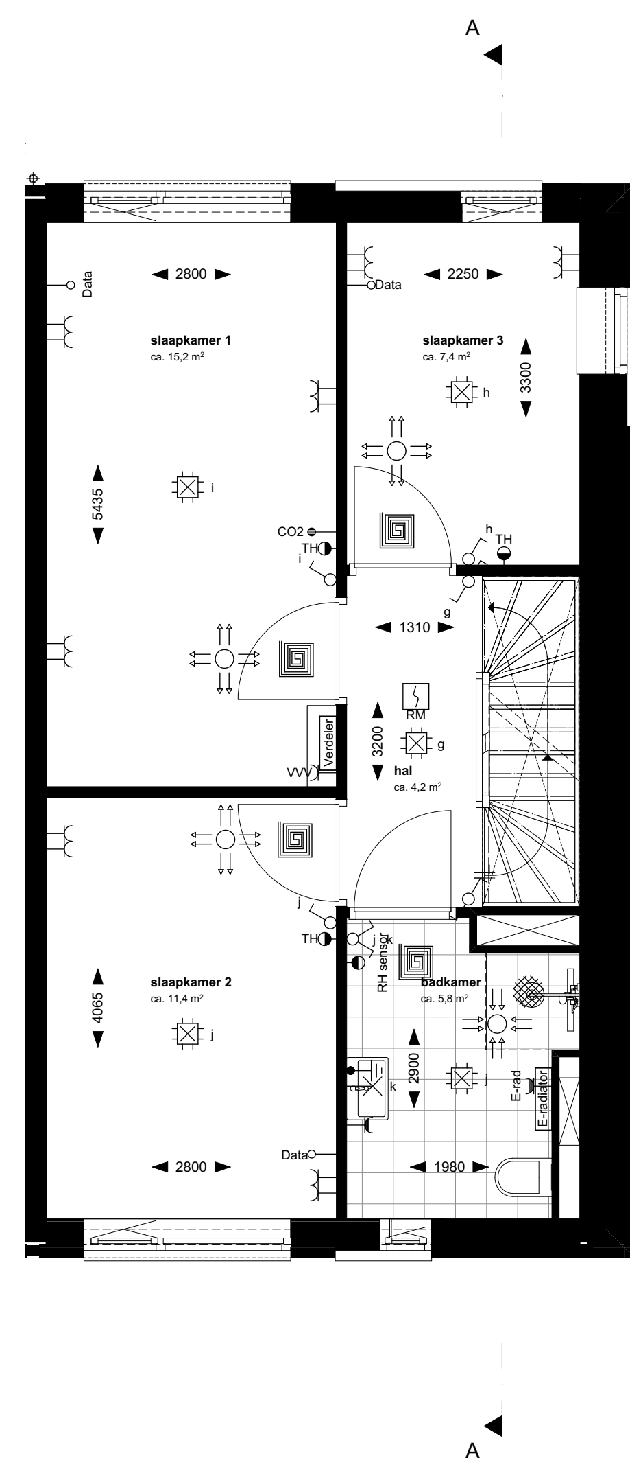
1E VERDIEPING
