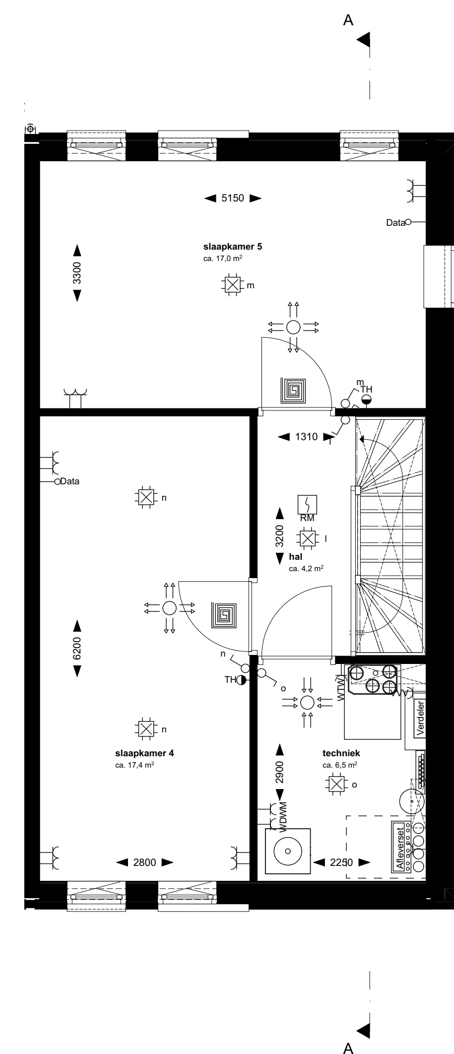
2E VERDIEPING
