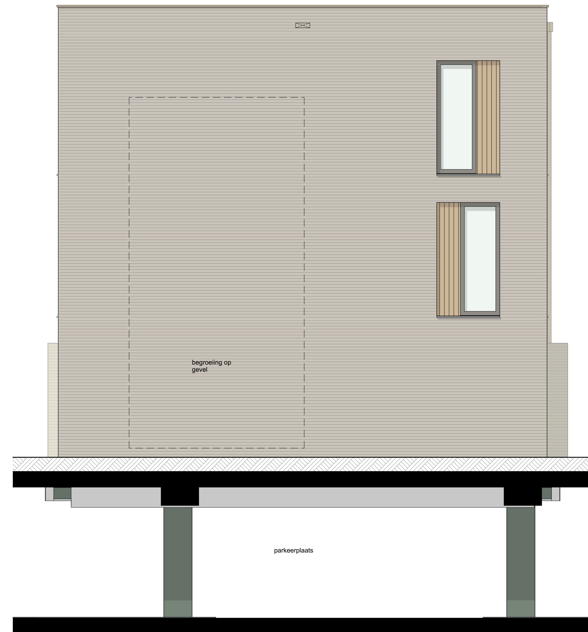
RECHTERGEVEL
